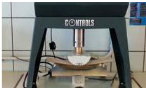
Измерение деформируемости цементных клеев
